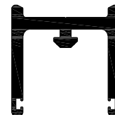
Befestigungsprofile
